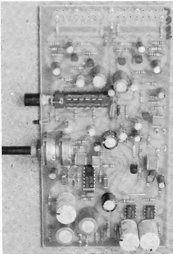
Koptelefoonmoduul
