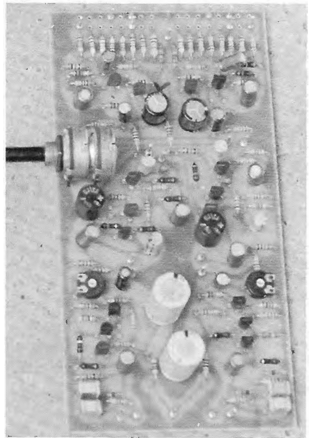
Lijnversterker/VU-metermoduul
